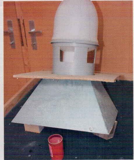
Von Rudolf Baswald entwickeltes Patent: Tränkenheizung mit Öl-Grablicht
